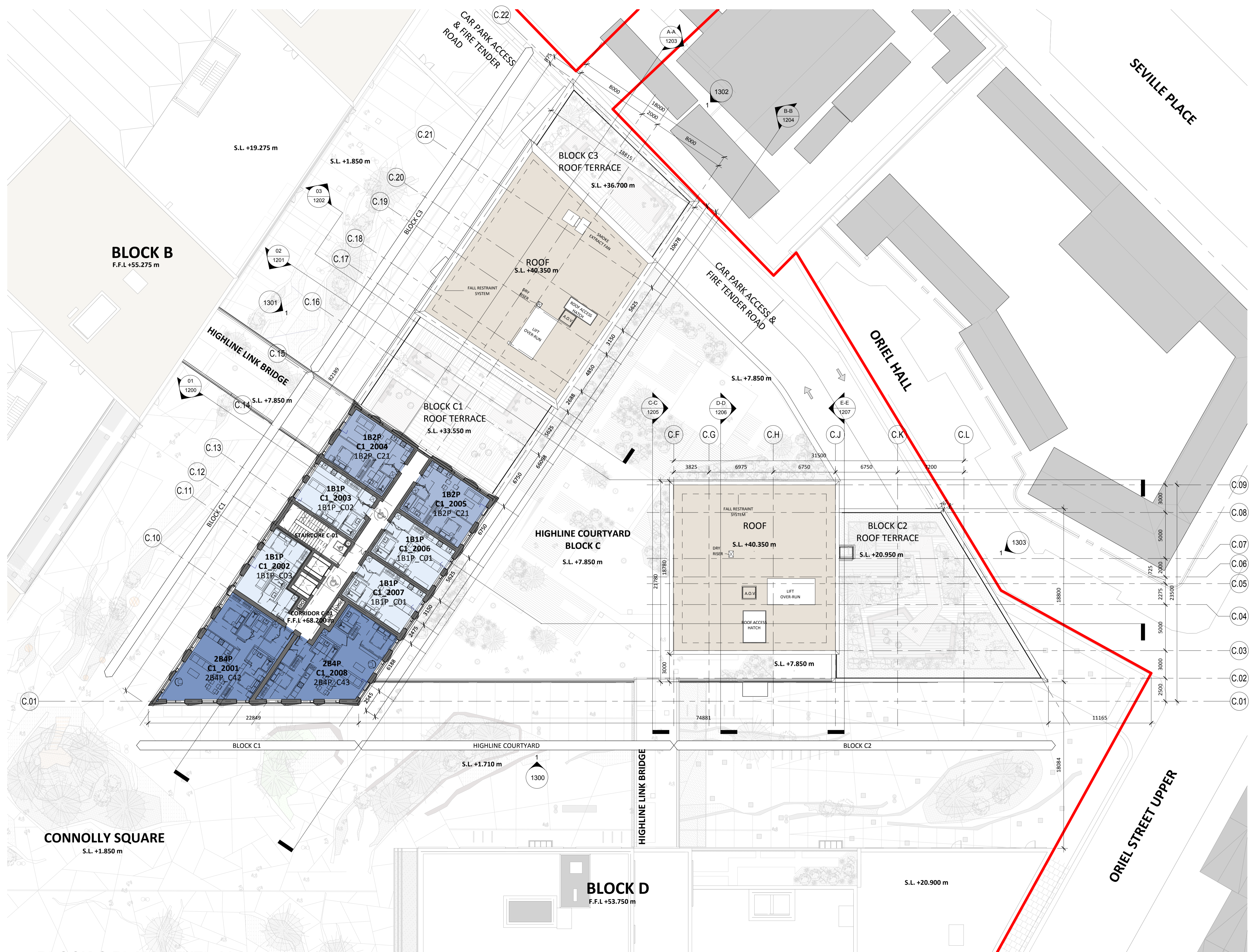
1 BLOCK C PLAN_LEVEL 20 1 : 200
